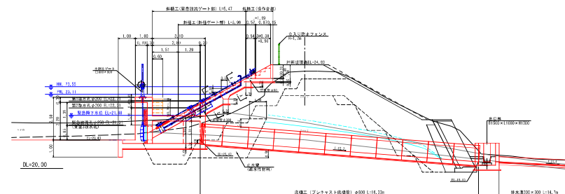
洪水吐工断面图
