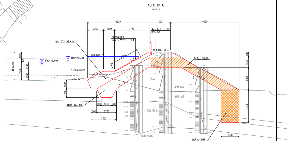
標準断面図
