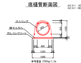
底槌管断面图
