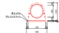
底樋工
