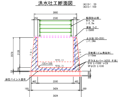
洪水吐工断面图
