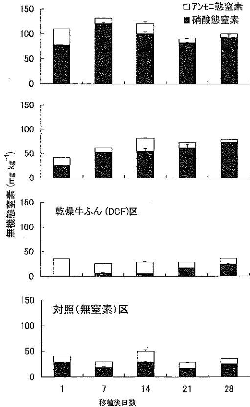
図7 栽培期間中の無作付け土壌の無機態窒素含量の推移(実験2) Vertical bars indicate standard error of mean (n=3).
