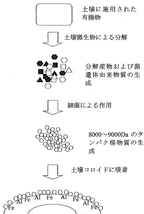
図25 土壤に施用された有機物が土壤固有の有機態窒素に取れんされるまでの模式図
