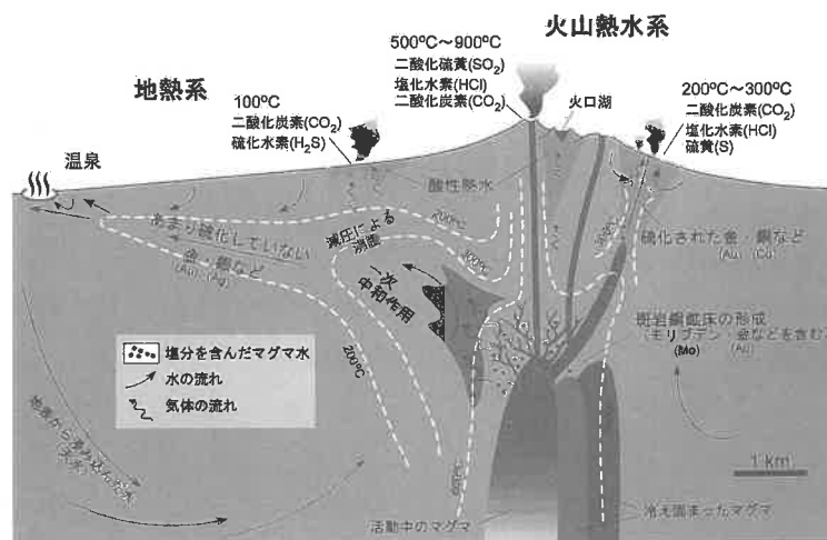
図 2-5-1 「マグマ熱水系モデル」における金の沈殿 (3)
