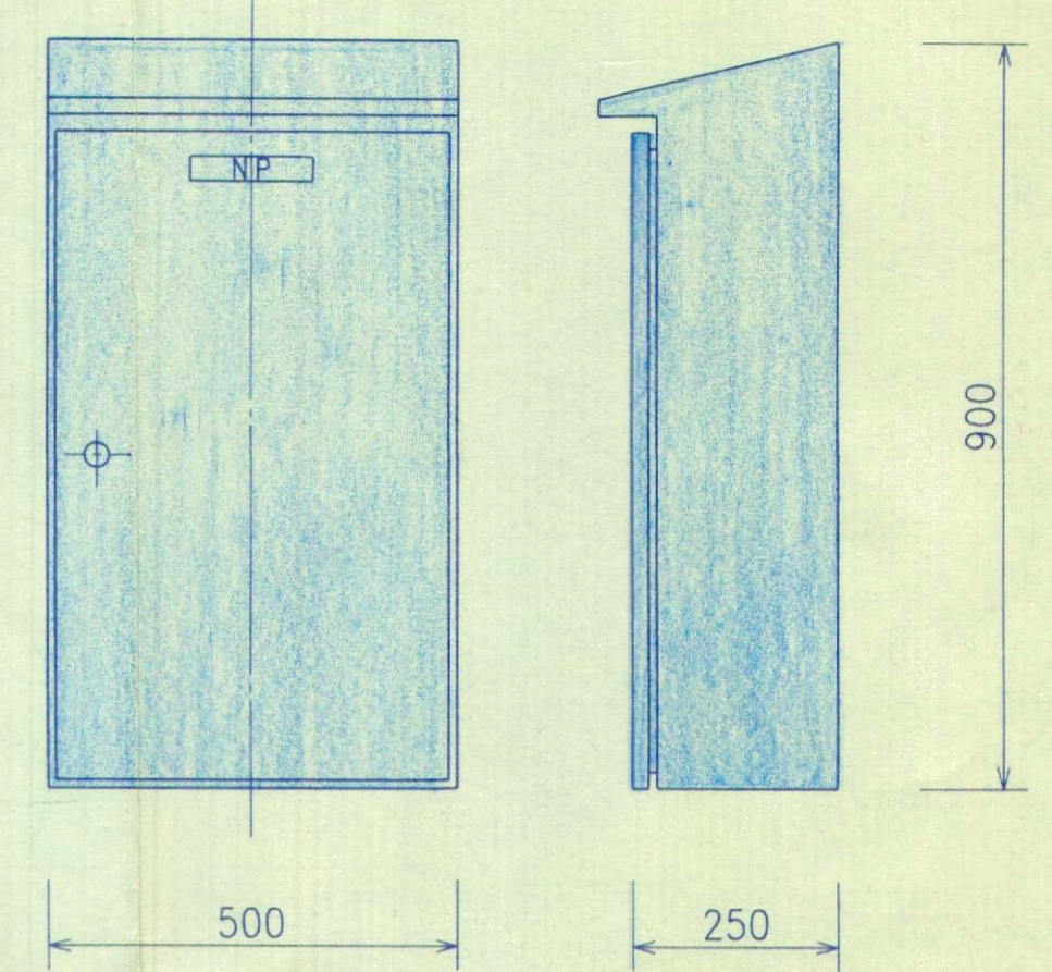
LA-14, LA-15 S=1:10 (下流ITV,上流ITV)
