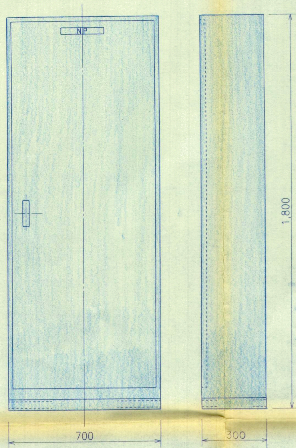
照明制御盤 LA-1 S=1:10 (電源室内)
