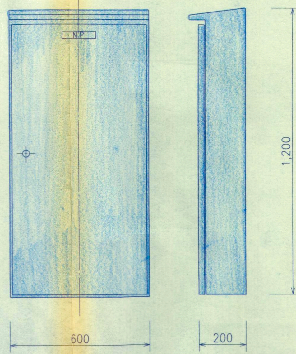
LB-1 S=1:10 (下流ライトアップ)
