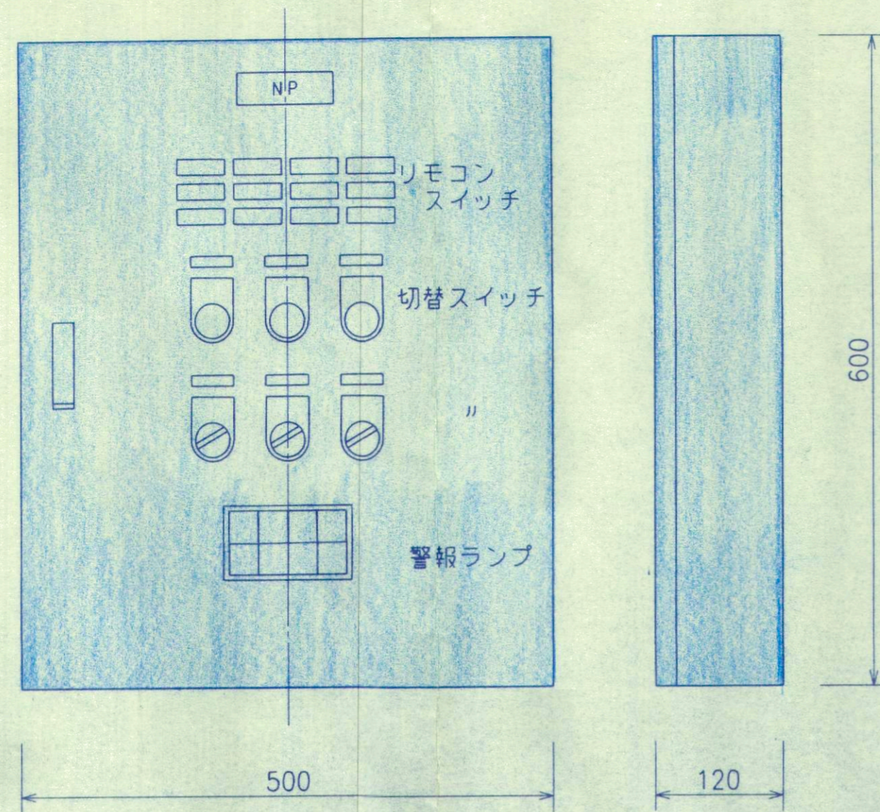
照明操作盤 LC-1 S=1:5 (管理所内)
