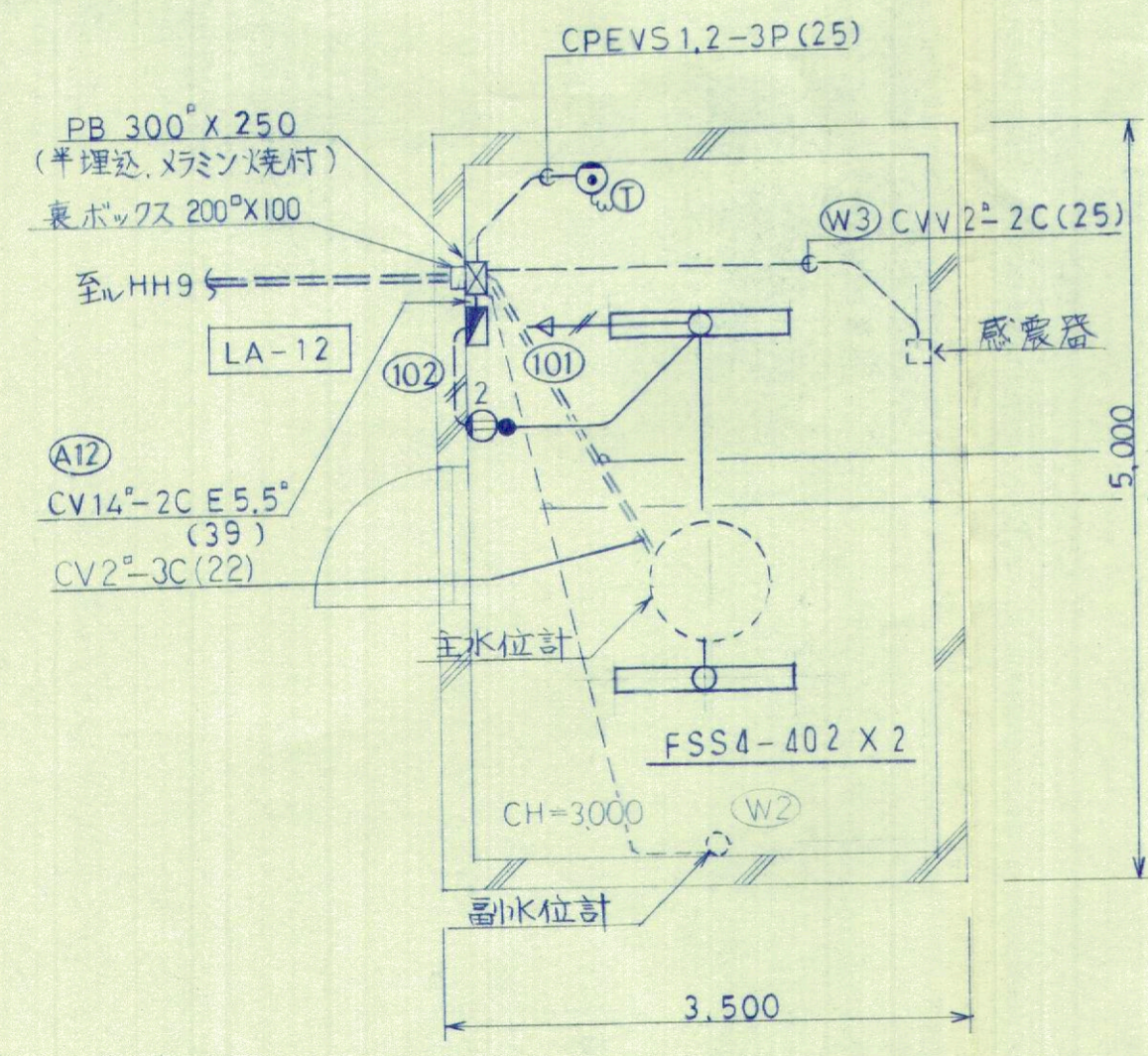
水位計室詳細図 S=1:50
