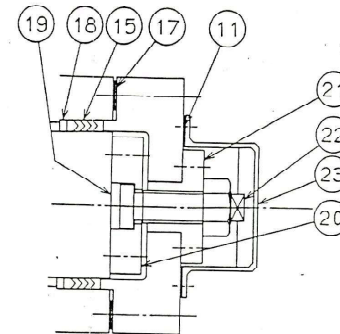
詳細 D
