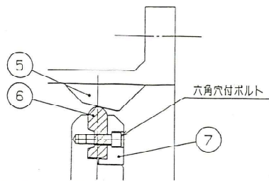
詳細 A
