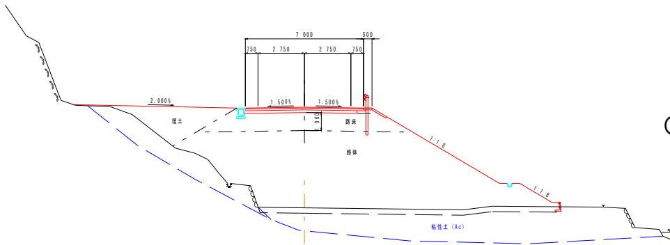
第2期工事 (盛土工事) 工期：R6.6～R7.2 予定
