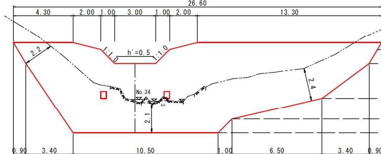
R5 (2工区) 1号谷止工
