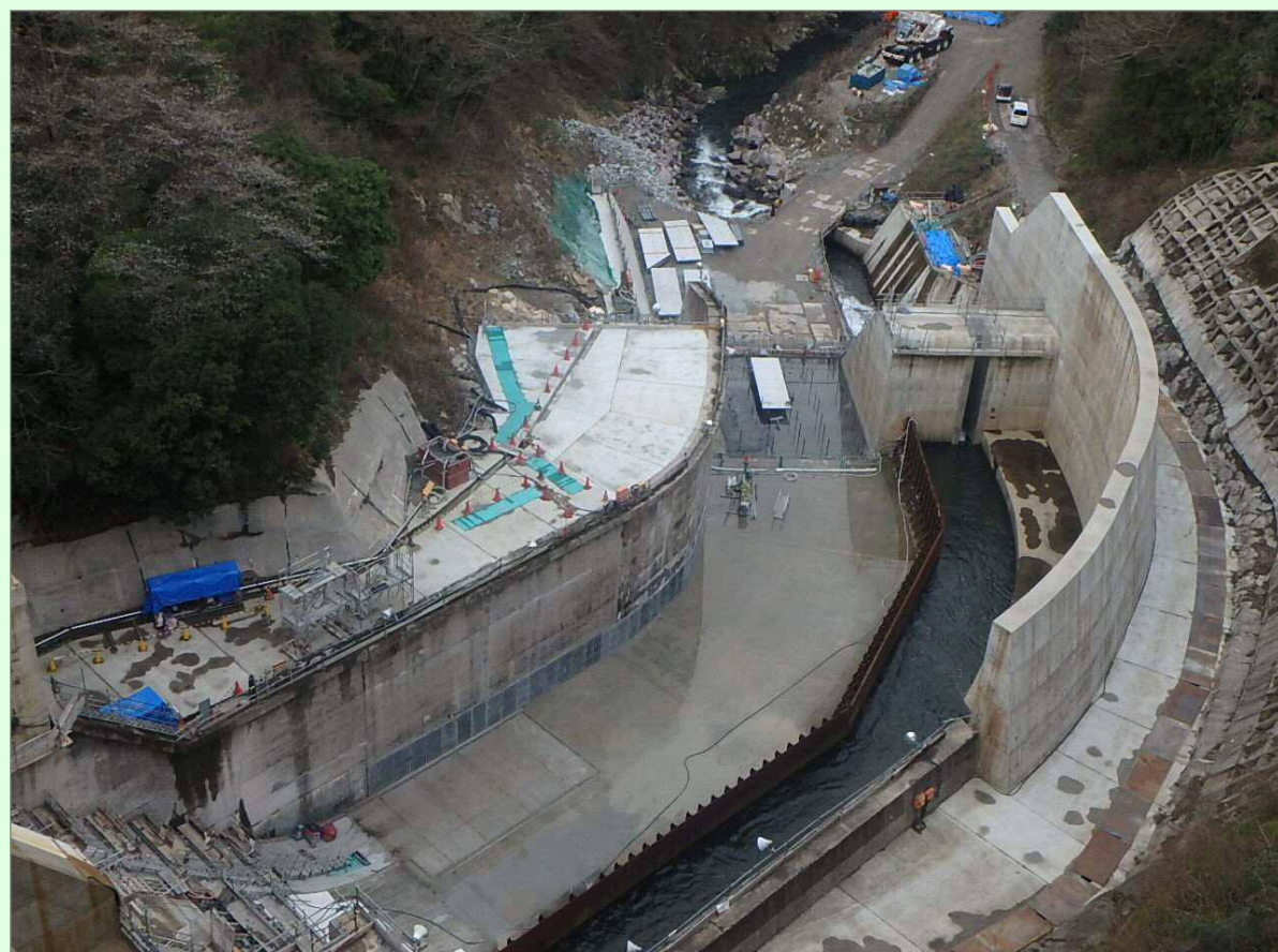
減勢工1
