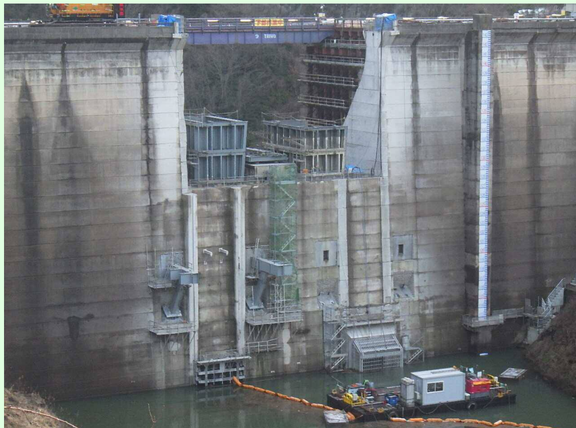
上流仮締切施工状況
