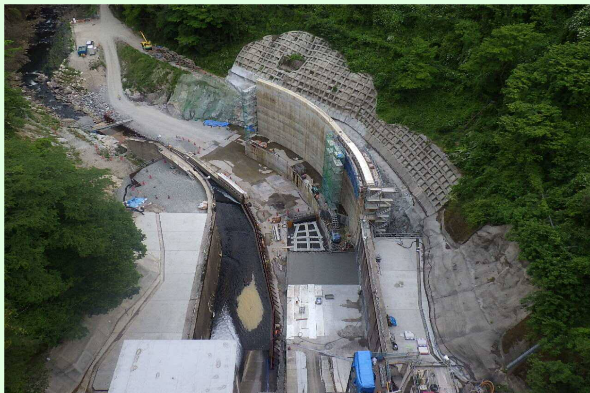
減勢工・工事用道路
