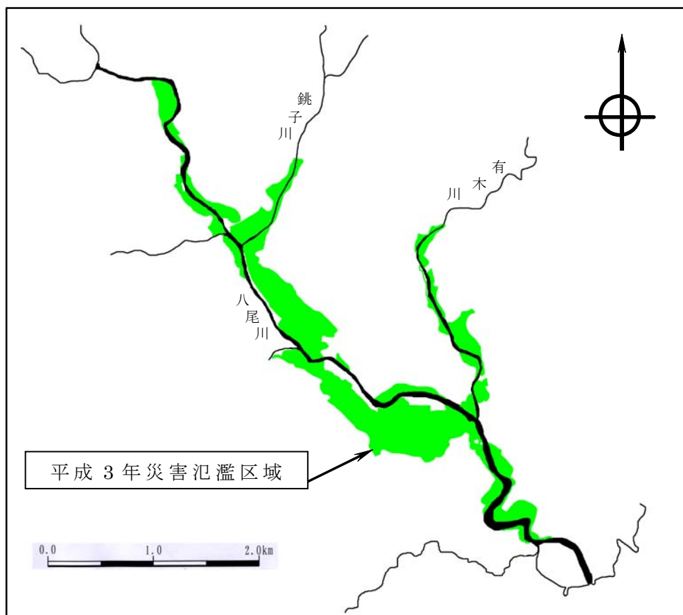
図1-2 氾濫区域図
