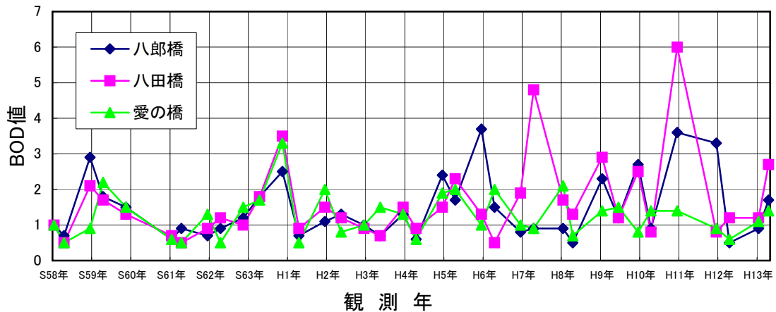
図 1-4 BODの推移
