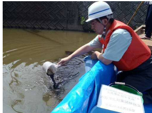
写真-3.3.12 水質浄化剤散布状況 （平成 26 年度）
