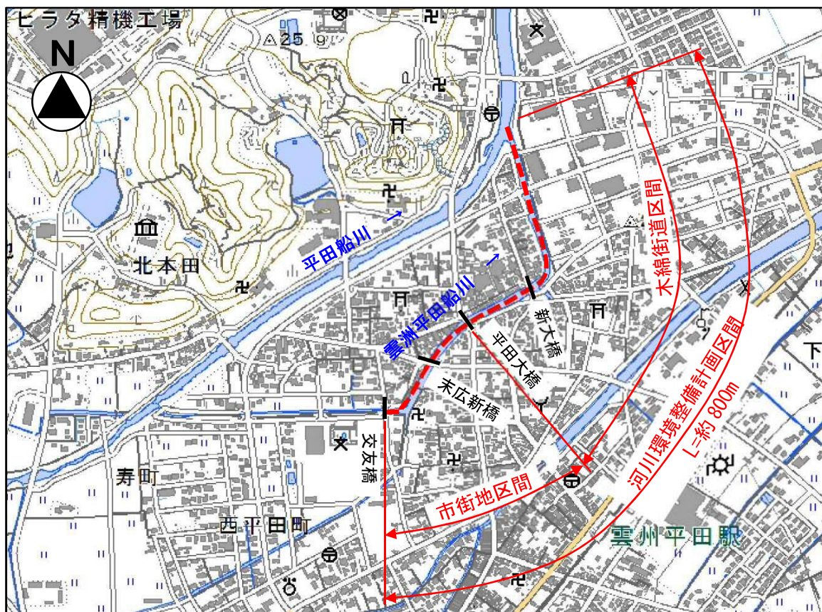
図-3.5.1 計画平面図
