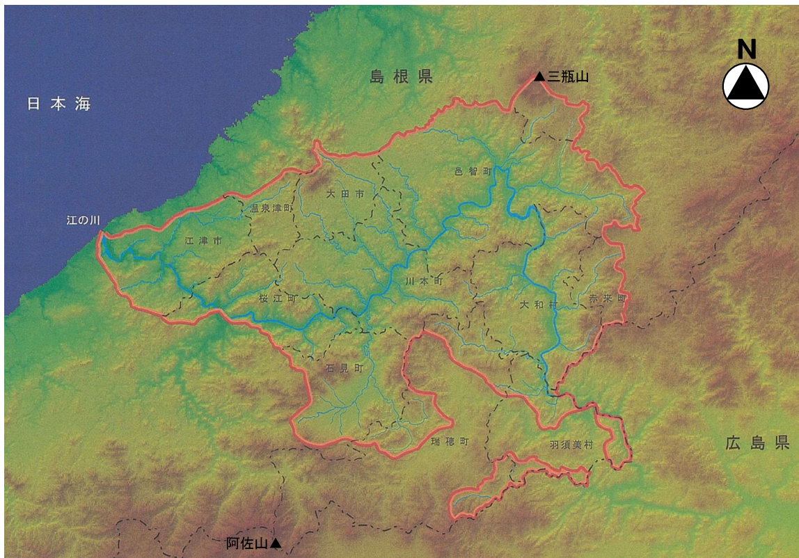
図 2-1 江の川水系下流支川域地形図
