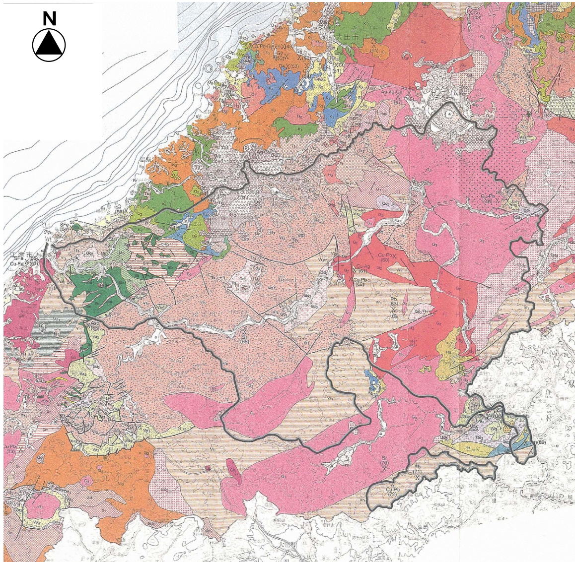
図 2-2 江の川水系下流支川域地質図
