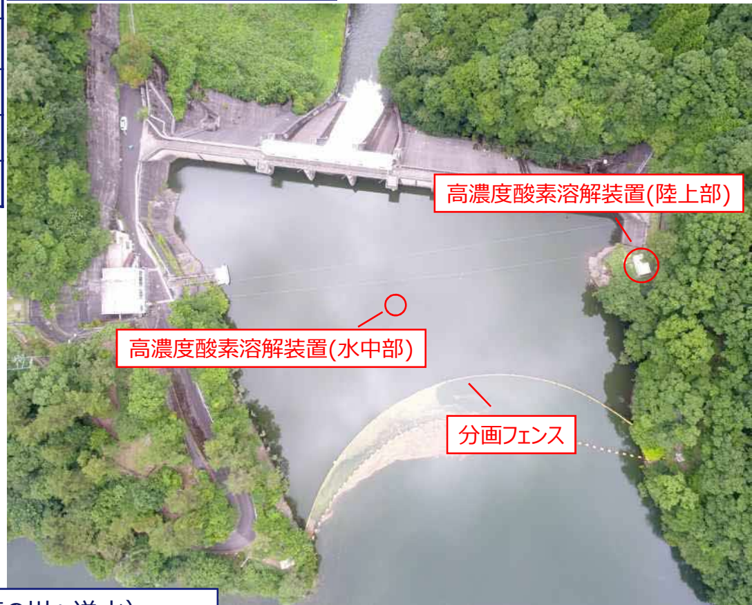
来島ダム水質保全設備
