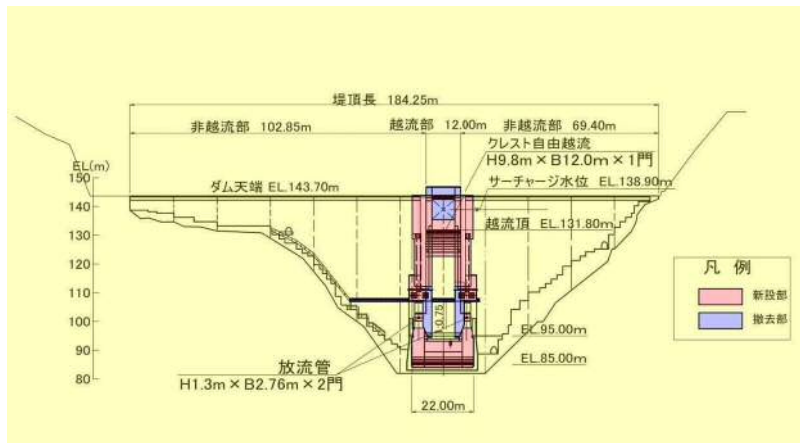
下流面図
