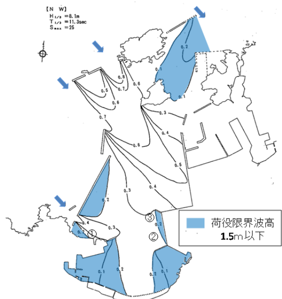
図 2-8 等波高比線図 (NW方向)
