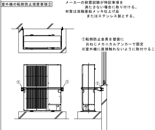
室外機の転倒防止措置要領②
