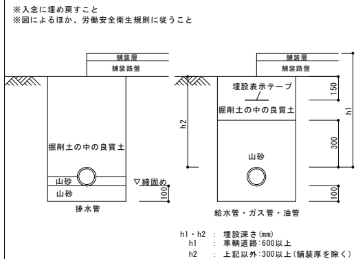
掘削基準断面図
