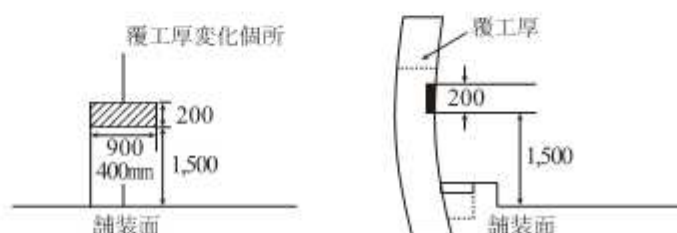
(取付け図)
