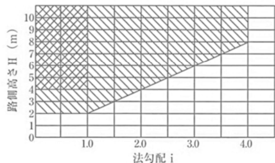
防護柵の設置基準・同解説(平成 20 年 1 月 31 日)
