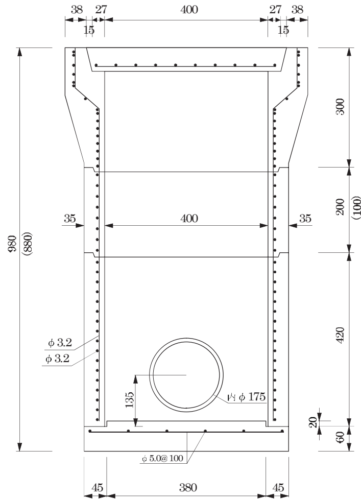
汚水樹図（遠心力鉄筋コンクリート）400型
