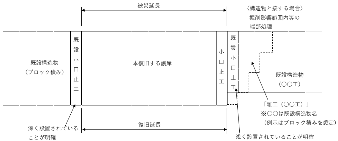
図－１ 既設小口止工の根入れ長が明確な場合
