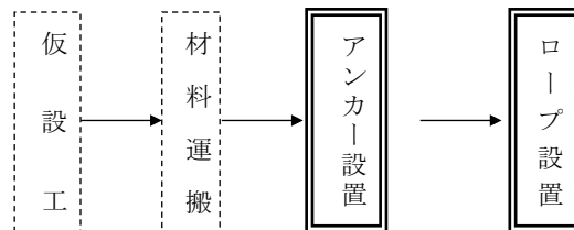
図2-1 施工フロー
