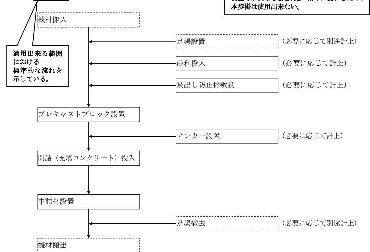
図1-1 施工フロー
