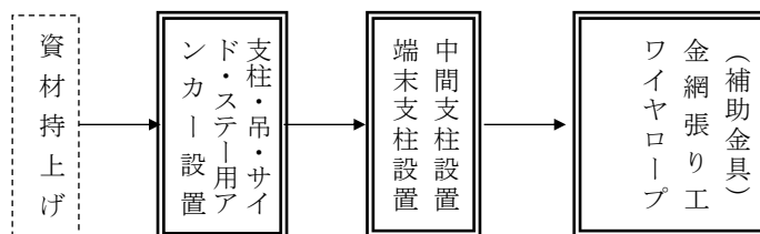
図2-1 施工フロー
