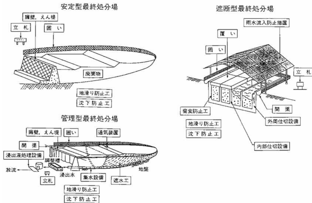
図一3 最終処分場概念図
