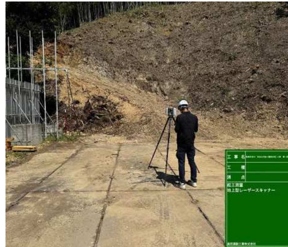
▲レーザースキャナーを使用した 起工測量
