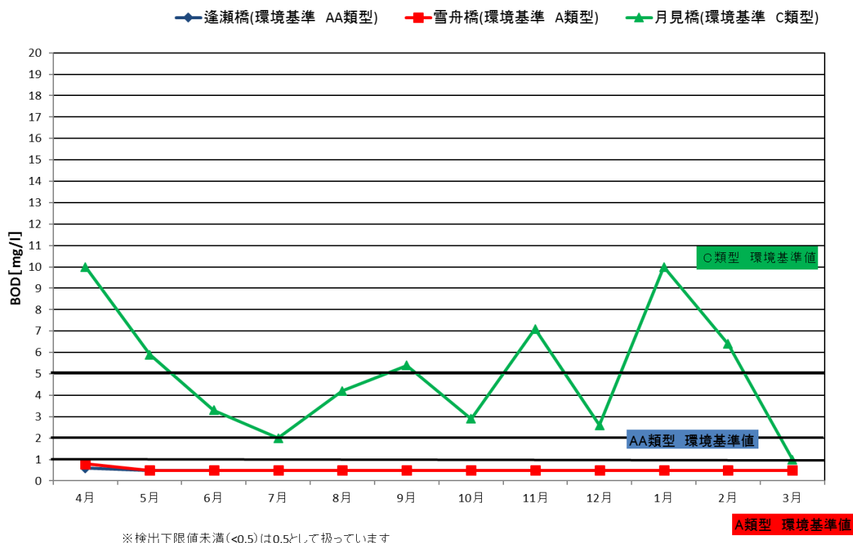
平成30年度益田川月別BOD変化(速報値)
