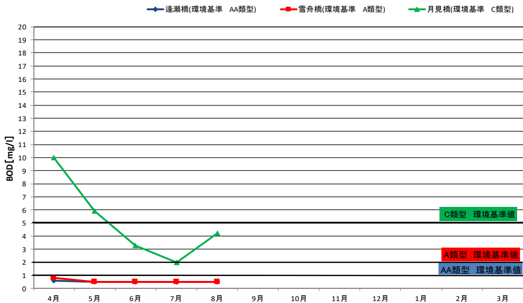
平成30年度益田川月別BOD変化(速報値)
