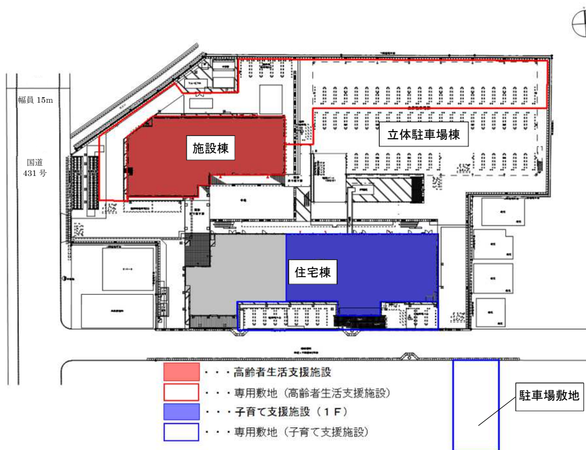
(2) 配置図
