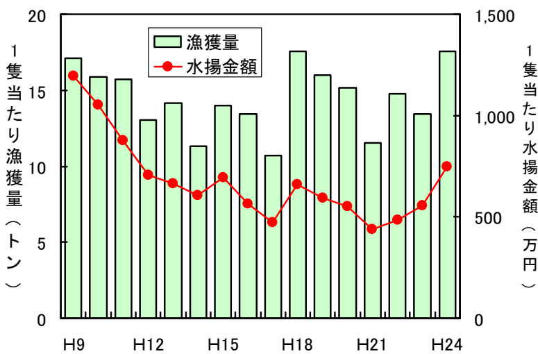
図 1 石見部および出雲部ばいかご漁業におけるエッチュウバイの 1 隻当たり漁獲量と水揚金額の推移
