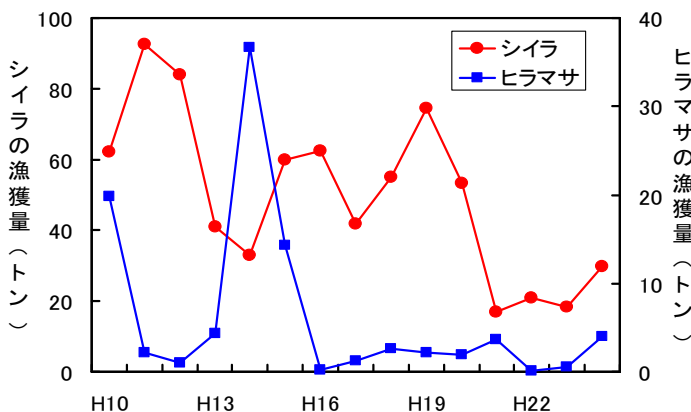
図4 シイラとヒラマサの1隻当たりの漁獲量の推移
