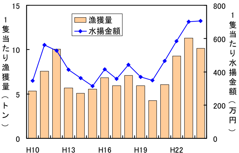
図 2 あなごかご漁業の 1 隻当たり漁獲量と水揚金額の推移
