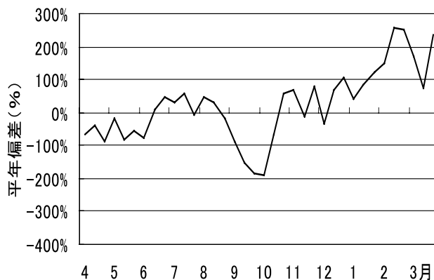
図5 恵曇港における表面水温の年偏差
