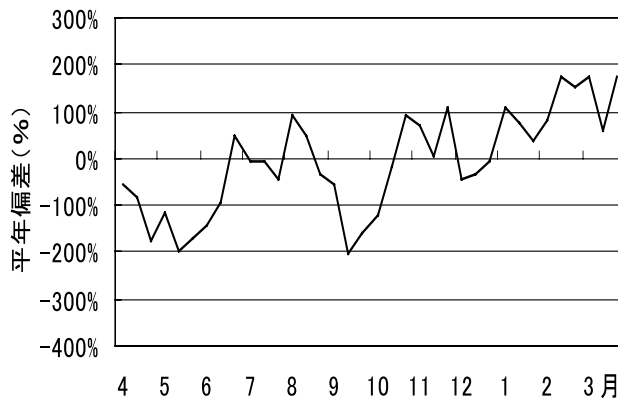
図3 浜田港における表面水温の年偏差
