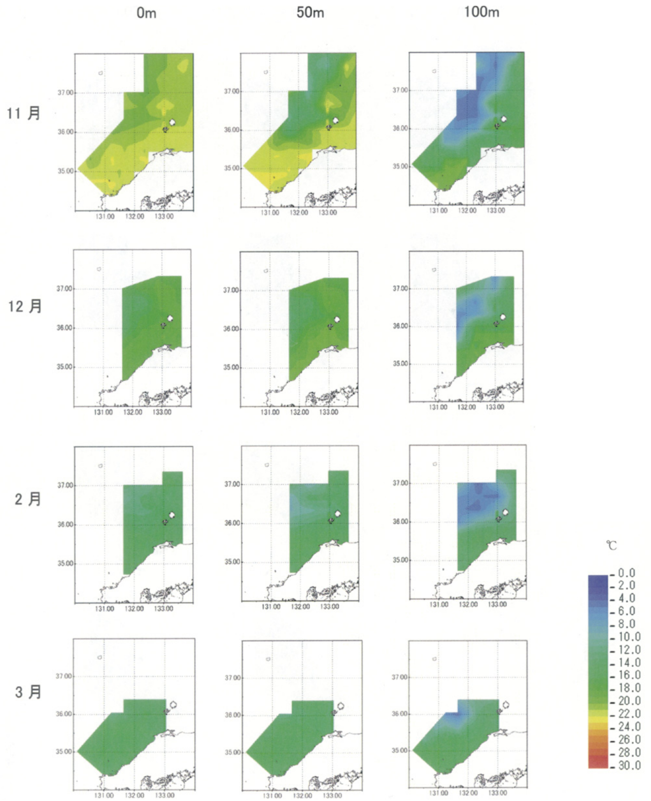
図 6-2 水温水平分布図 (11～3 月)
