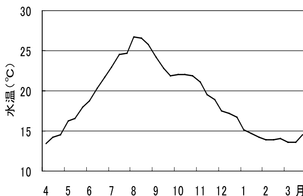
図4 恵曇港における表面水温の旬平均
