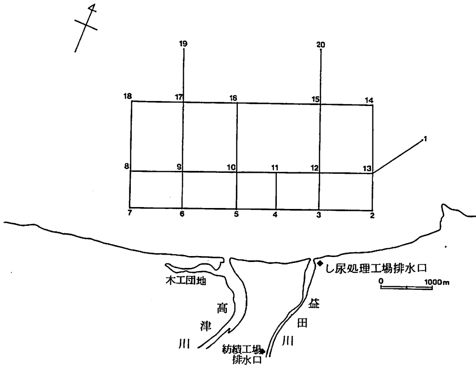
図1 益田地先調査定点配置図
