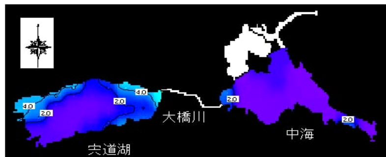
底層における塩分分布 (2001年8月)
