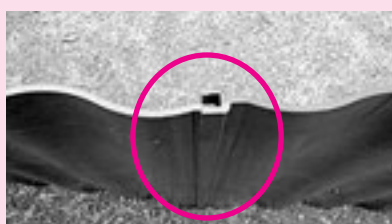
上段: 波板の継ぎ目から侵入する地下茎 (手前側を掘り起こして撮影) 下段: 継ぎ手で結合できる資材 (畦板)
