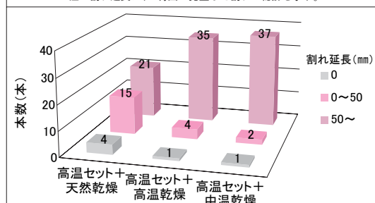
図2 内部割れによる品質区分結果
