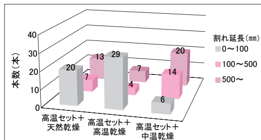
図1 材面割れによる品質区分結果
