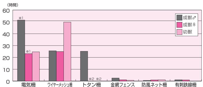
図1 各侵入防止柵を突破するまでの時間 （※1 電気ショックに驚いて突破。※2 成獣♂の突破によって破損したために計測不能）
