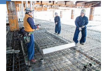
【鋼製型枠を鉄筋上に取付けている作業風景（左が外国人材）】
