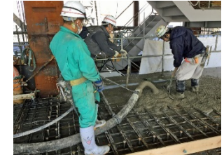
【圧送ポンプを利用して型枠内にコンクリートを打ち込むところ】
