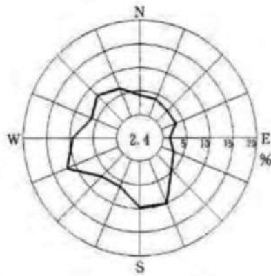
標高 65 m (地上高 50 m)
