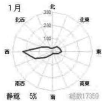
図1-1 松江地方気象台
