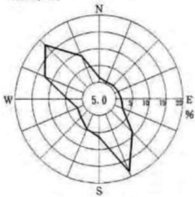
標高 28.5 m (地上高 20 m) 1996年7月
