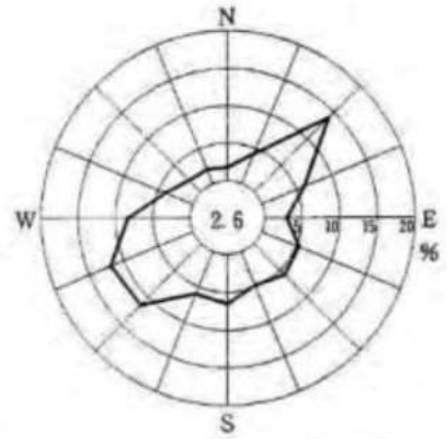
標高 130 m (地上高 115 m)
