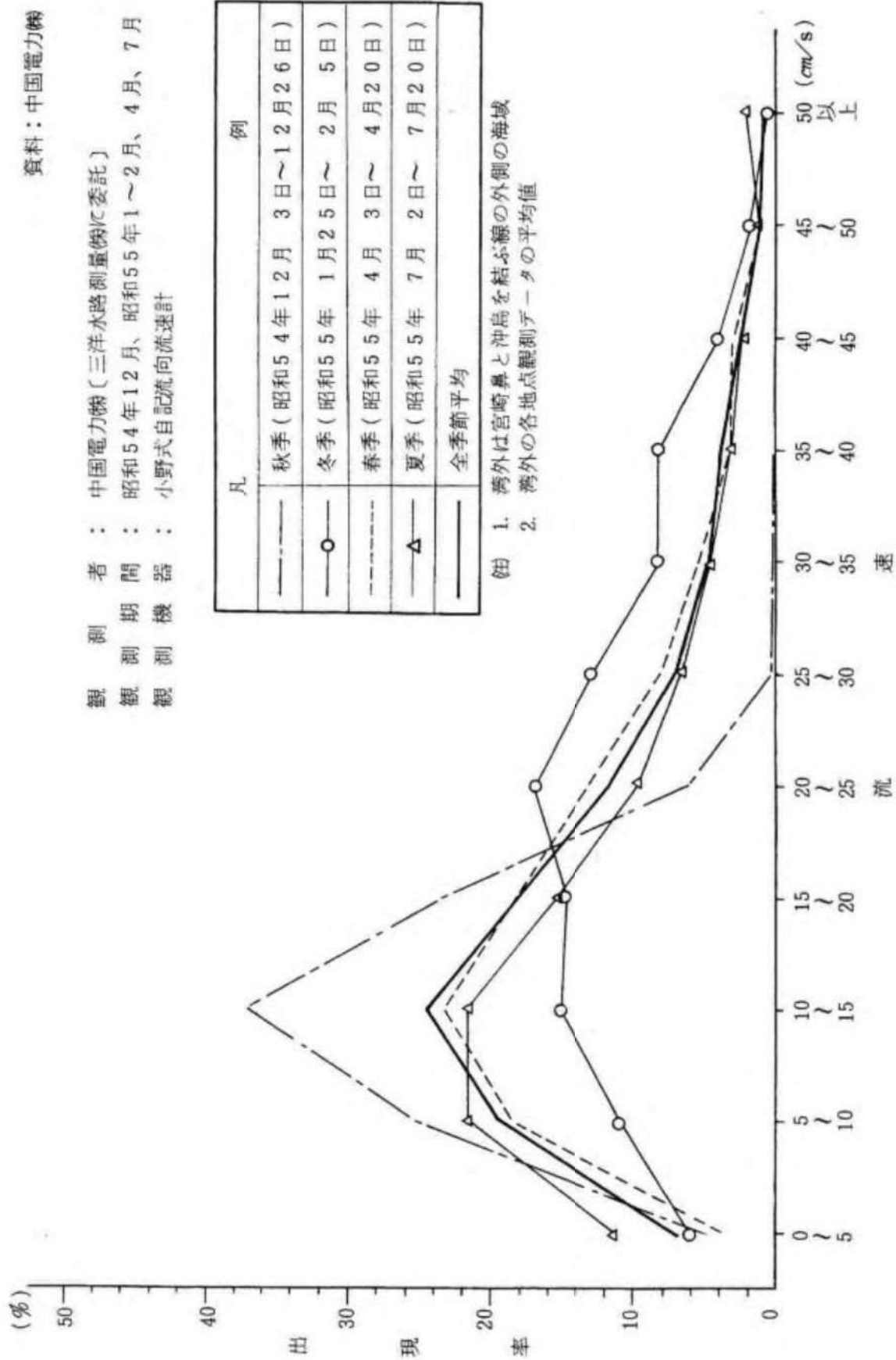
湾外の流速別出現頻度図 (四季)
