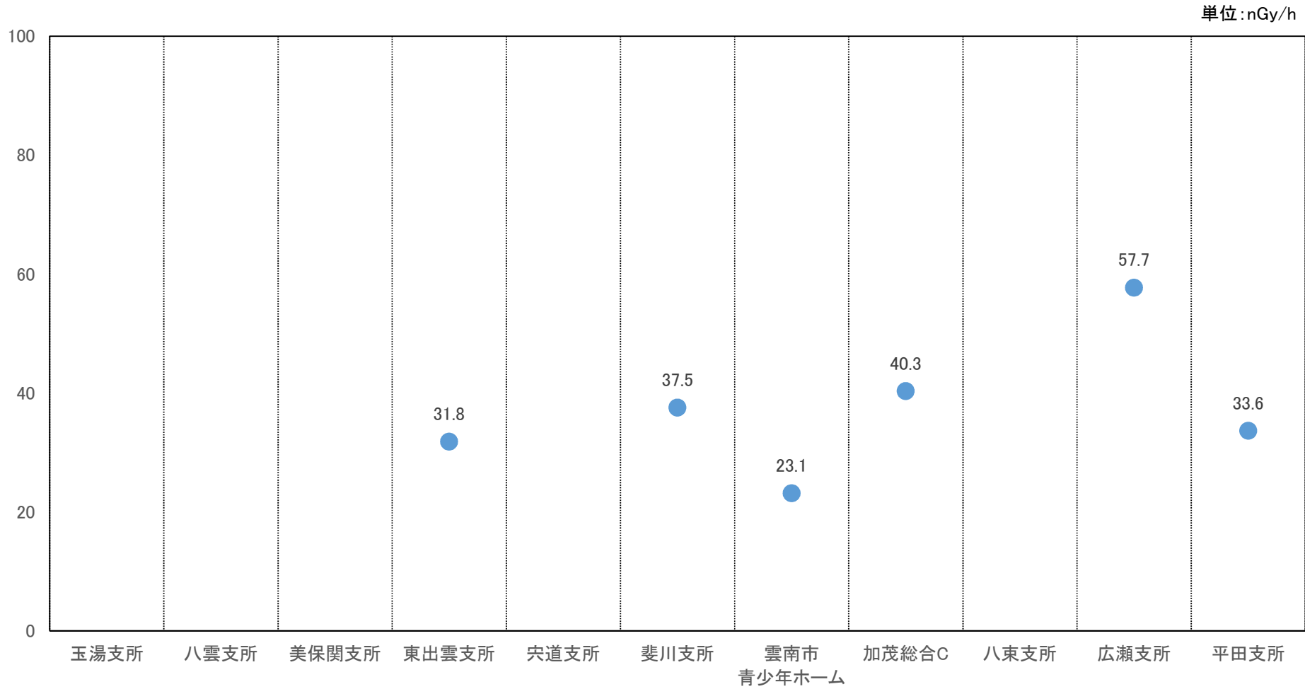
可搬型モニタリングポスト:速報値 令和2年5月18日～5月24日における空間放射線量率(平均値)
