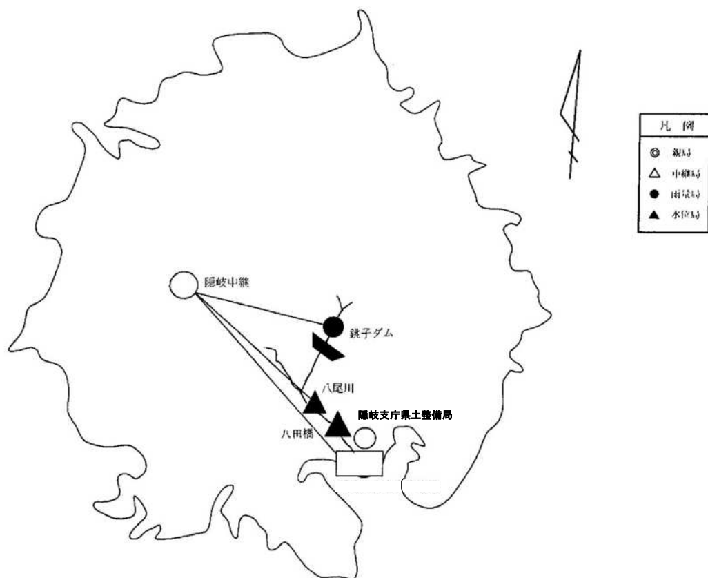
Q-2 図(40) 銚子ダムテレメーター回線系統図 (島根県)
