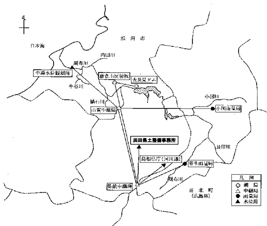
K-2図(28) 大長見ダムテレメーター回線系統図（島根県）
