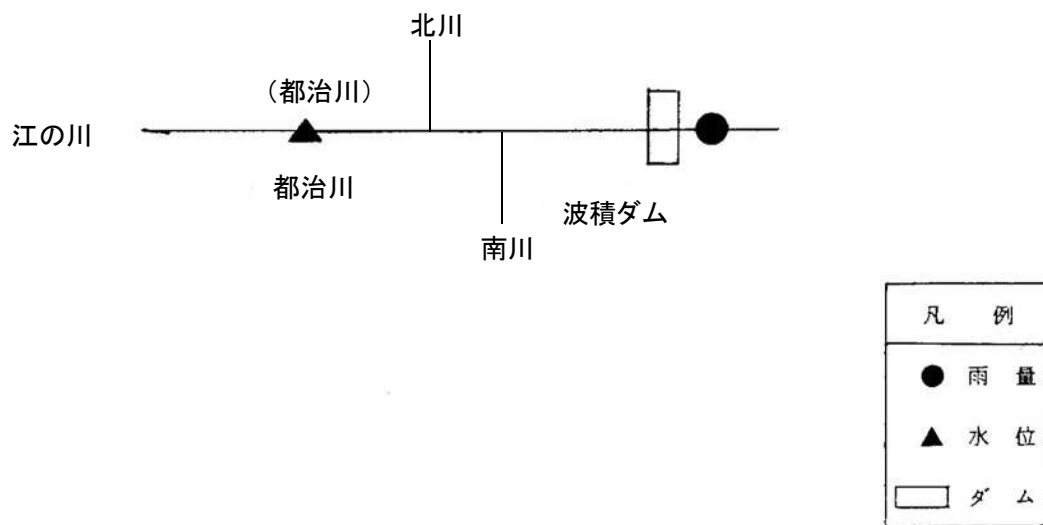
I-1 図(23) 波積ダム流域観測地点（島根県テレメーター）
