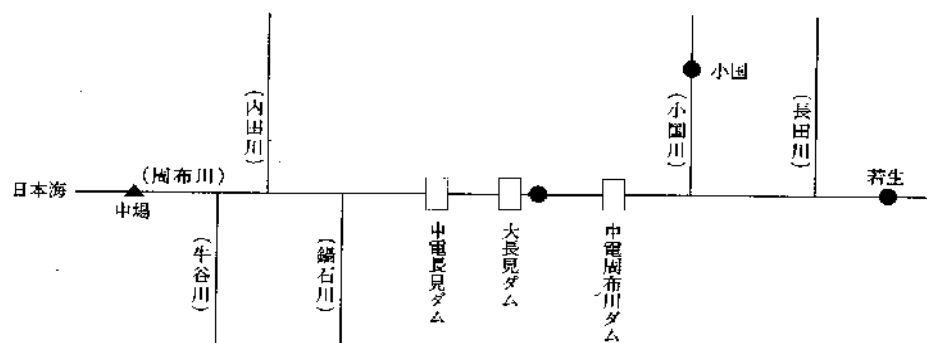
K-1図(27) 大長見ダム流域観測地点（島根県テレメーター）
