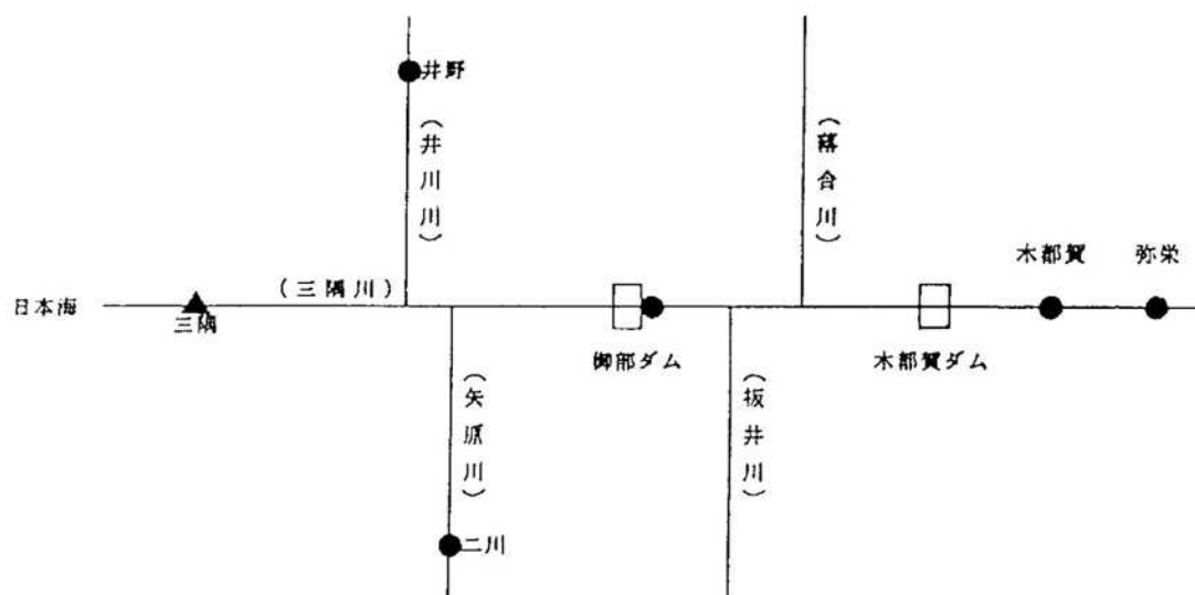
L-1 図(29) 御部ダム流域観測地点（島根県テレメーター）
