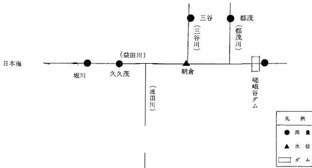
N-1 図(3 3) 益田川水系流域観測地点 (島根県農地テレメーター)
