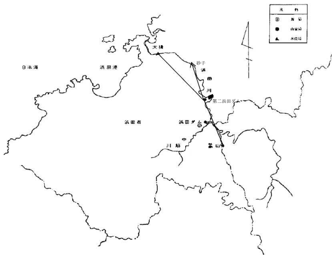
J-2 図(26) 第二浜田ダムテレメーター回線系統図（島根県）
