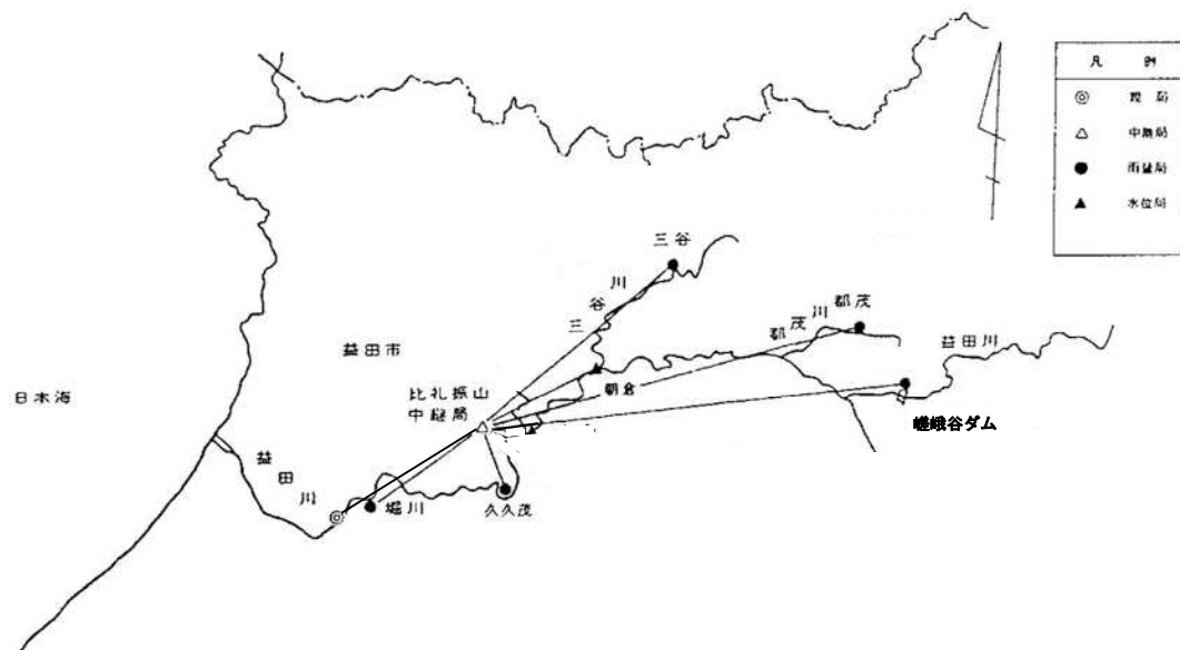
N-2 図(3 4) 益田川水系テレメーター回線系統図 (島根県農地)
