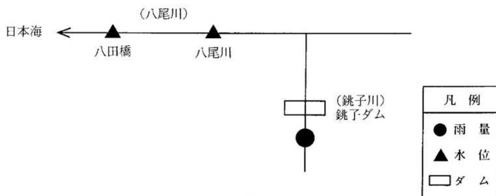
Q-1 図(39) 銚子ダム流域観測地点 (島根県テレメーター)
