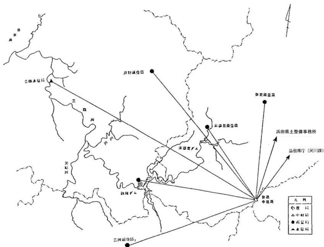
L-2 図(30) 御部ダムテレメーター回線系統図（島根県）
