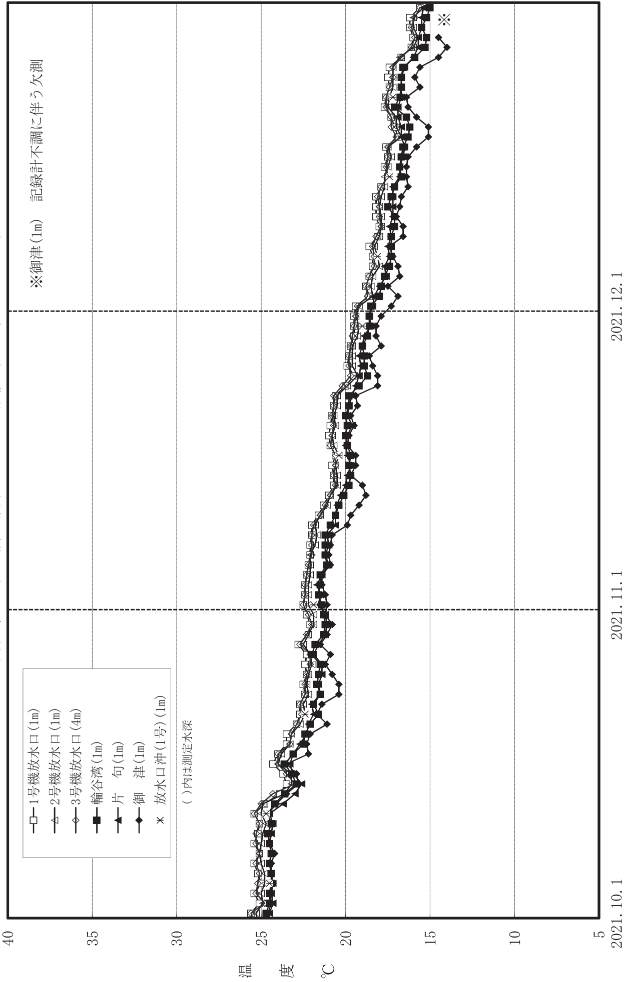
島根原子力発電所 沿岸定点の水温推移 (2021年10月~12月)
