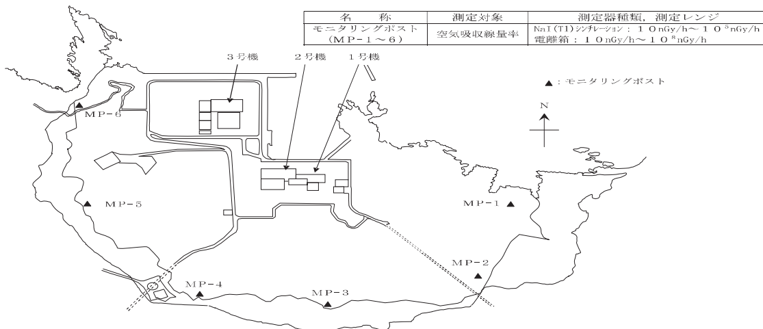
発電所敷地周辺の放射線測定設備
