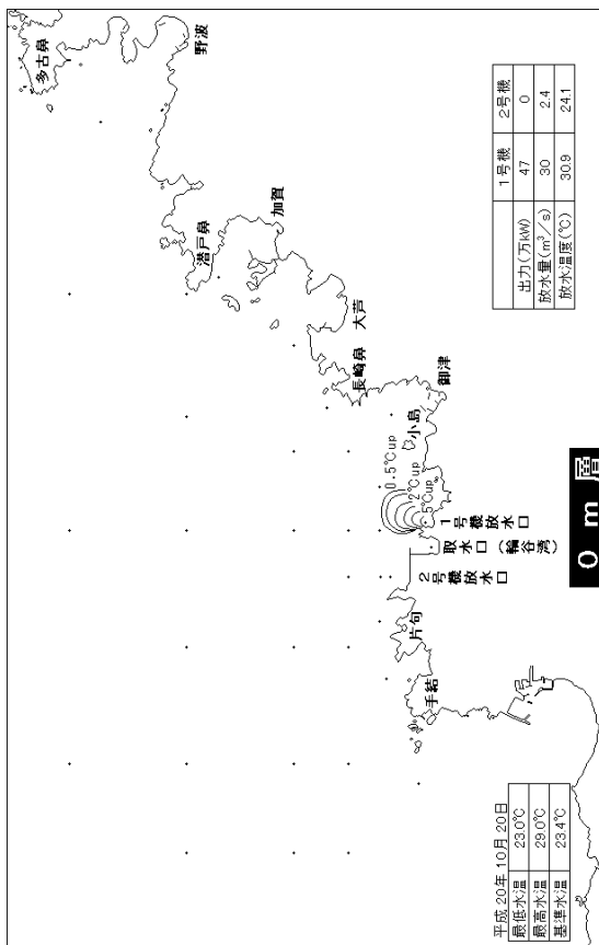
島根原子力発電所 沖合定線の水温水平分布図 (基準水温との温度差) 平成20年10月20日
