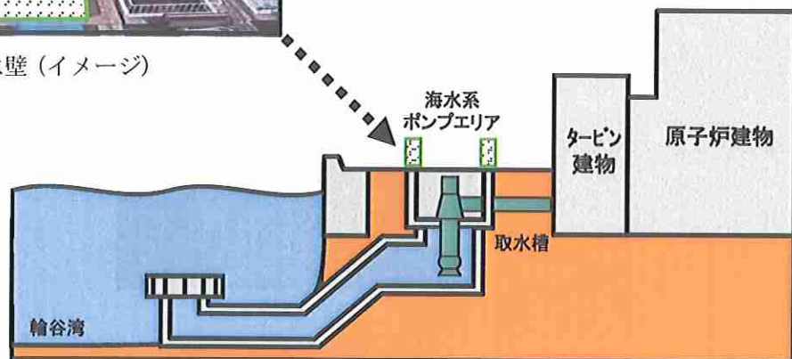
【海水系ポンプエリアの浸水防止対策イメージ図】
