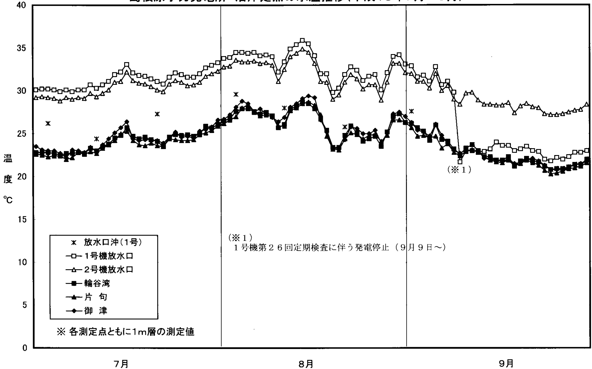
島根原子力発電所 沿岸定点の水温推移(平成18年7月~9月)
