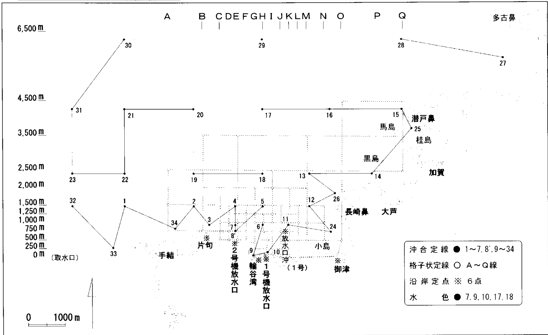
付図3 温排水測定地点図
