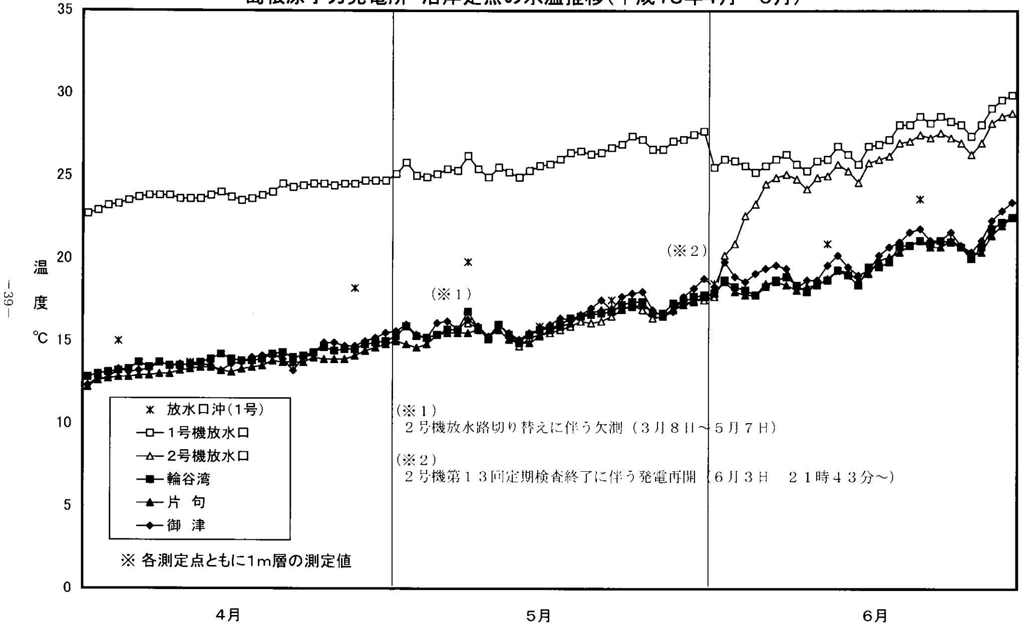
島根原子力発電所 沿岸定点の水温推移(平成18年4月～6月)
