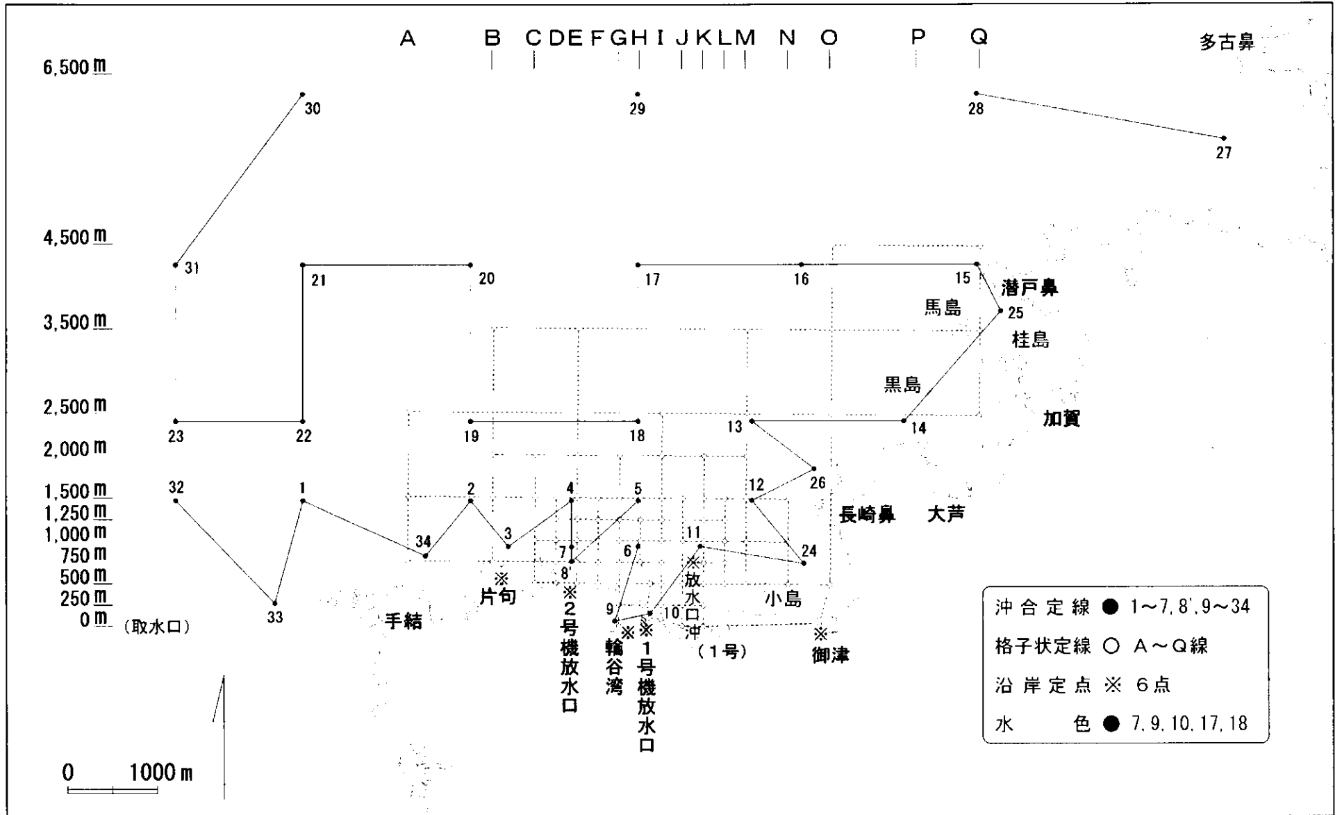
付図3 温排水測定地点図
