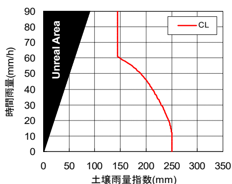
35331102(RBFN出力値0.2)
