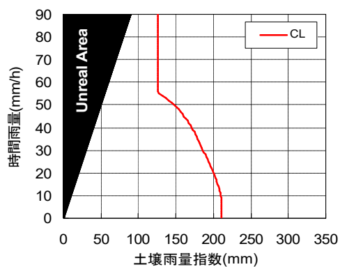
35330202 (RBFN出力値0.4)
