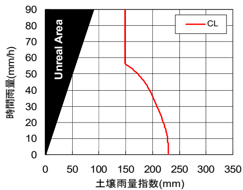
34311212(RBFN出力値0.2)
