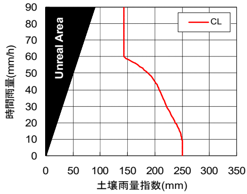
35320003 (RBFN出力値0.2)
