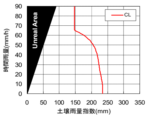
34321705(RBFN出力値0.2)
