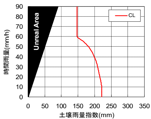
34321605(RBFN出力値0.2)
