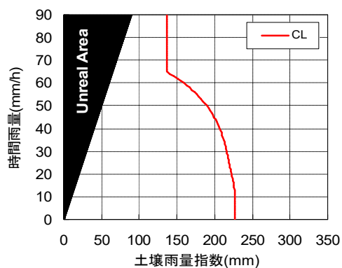
35320612(RBFN出力値0.2)
