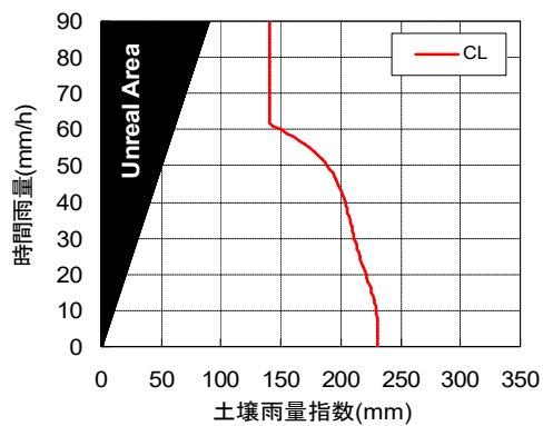
35320713 (RBFN出力値0.2)
