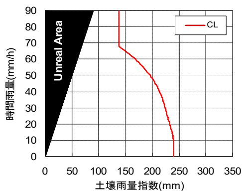
35320309(RBFN出力値0.2)
