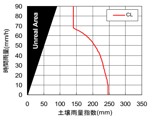
35320209(RBFN出力値0.2)
