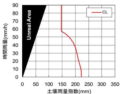
34321700 (RBFN出力値0.2)
