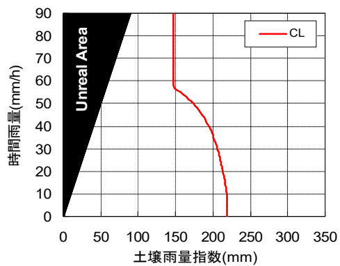
34321706(RBFN出力値0.2)
