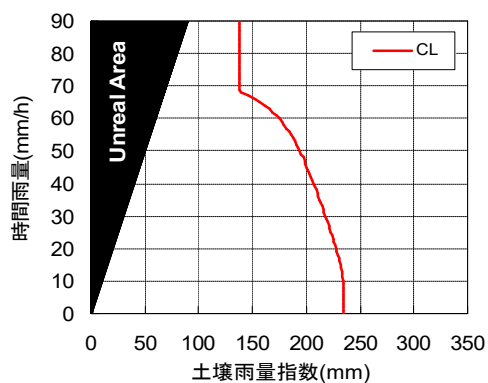
35320308(RBFN出力値0.2)
