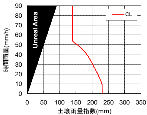
35330403 (RBFN出力値0.2)
