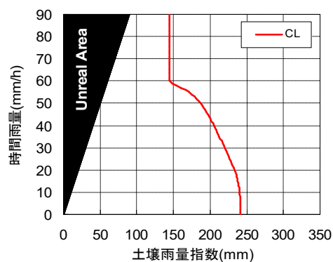
35321014(RBFN出力値0.2)
