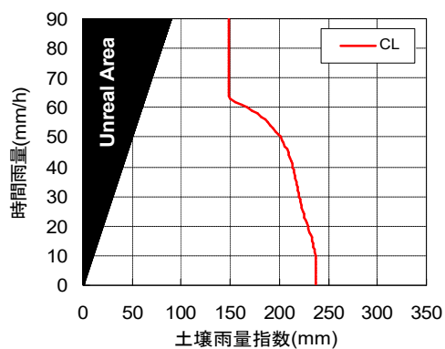
34311311(RBFN出力値0.2)
