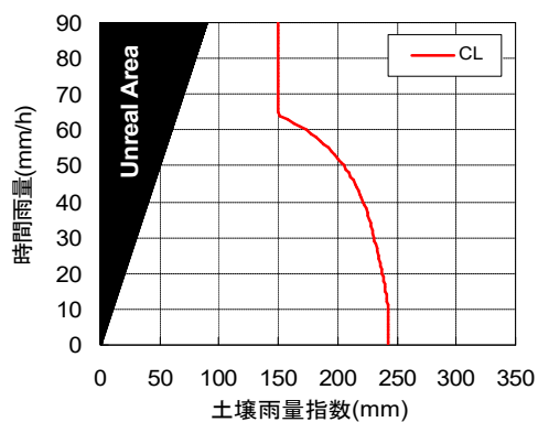
34310814 (RBFN出力値0.2)
