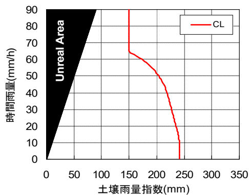
34310915 (RBFN出力値0.2)
