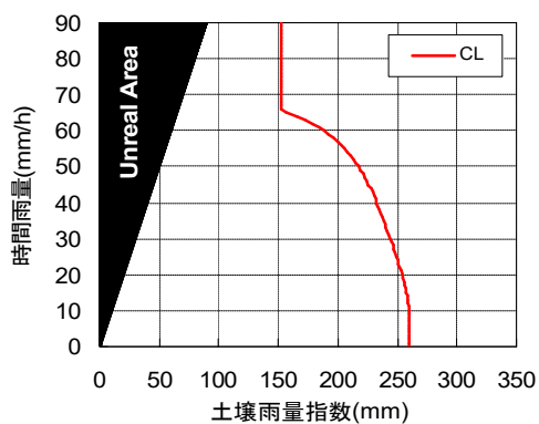
34310811(RBFN出力値0.2)
