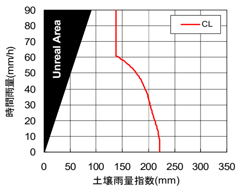
35320509(RBFN出力値0.2)
