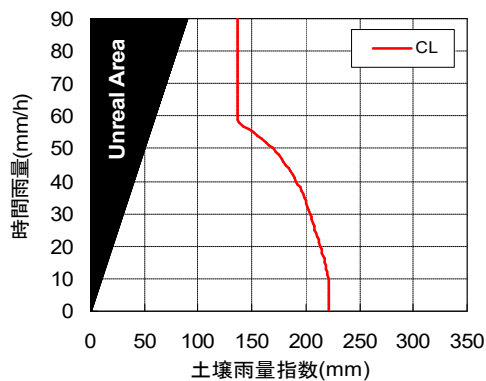
35320811 (RBFN出力値0.2)
