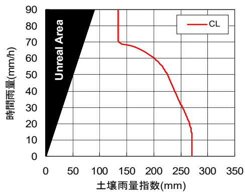
34321506 (RBFN出力値0.2)
