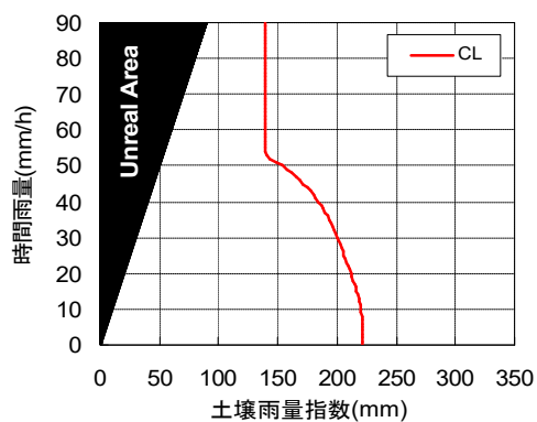
35330504 (RBFN出力値0.2)
