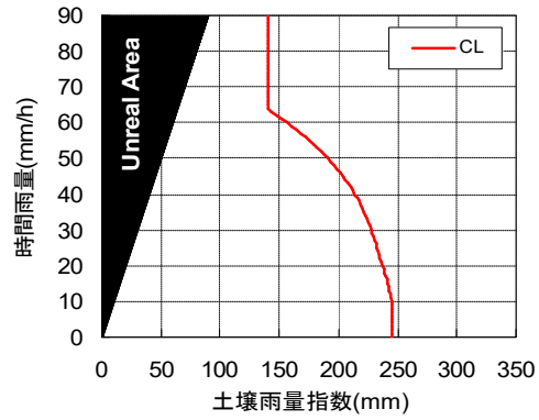
35320214(RBFN出力値0.2)
