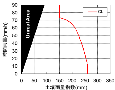
34310614 (RBFN出力値0.2)
