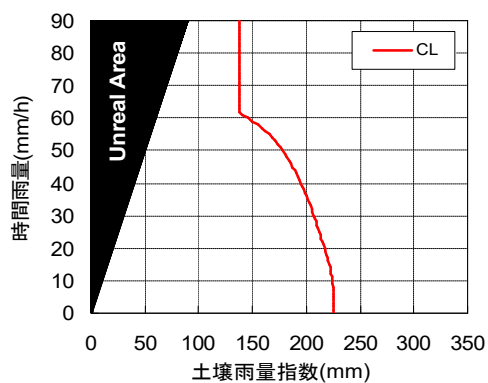
35320409(RBFN出力値0.2)
