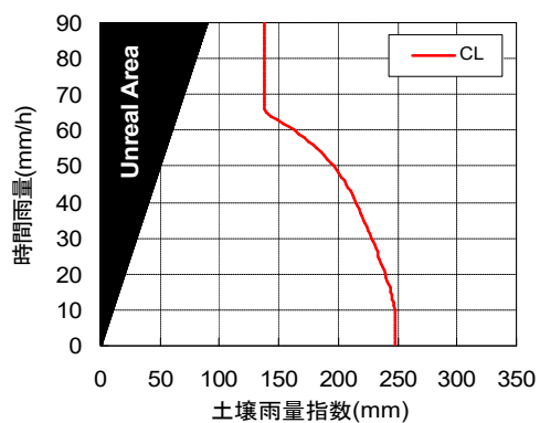
35320310(RBFN出力値0.2)
