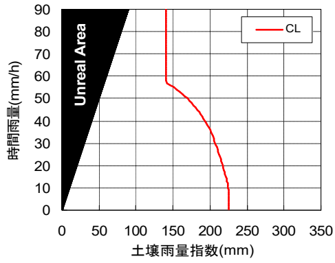
35320513(RBFN出力値0.2)
