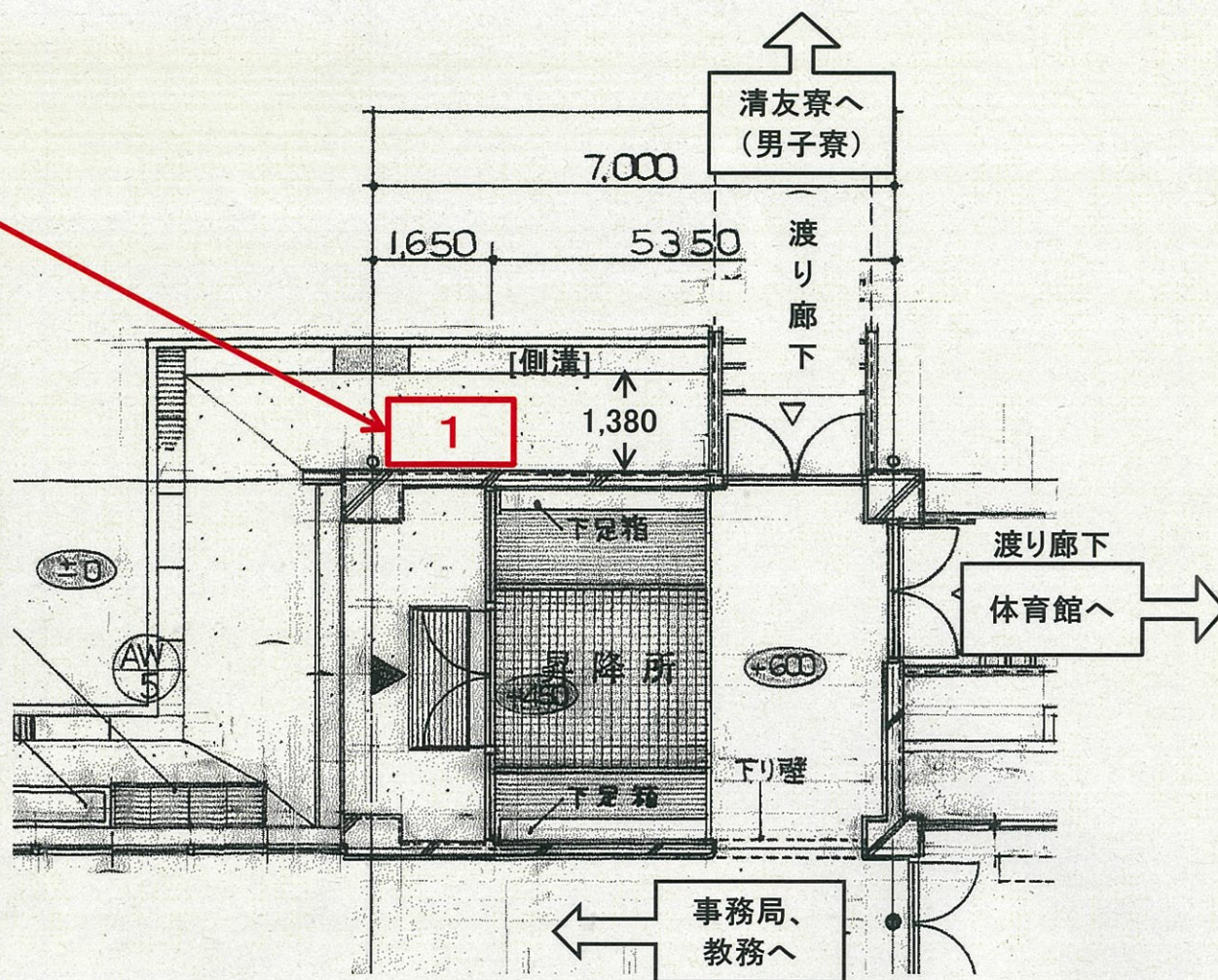
1階 平面図
