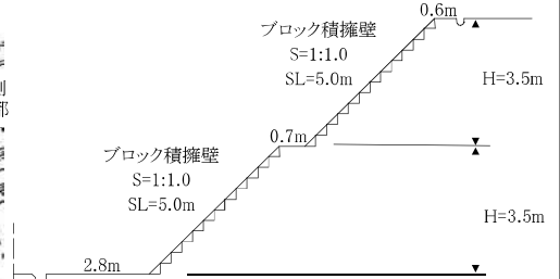
概略断面図
